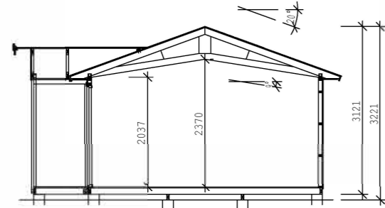
SEKTION
