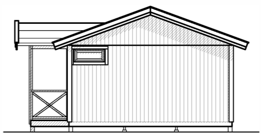
FASAD MOT
